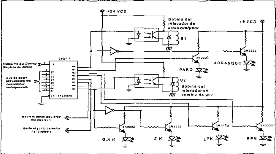
Figura 4.20. Circuito de salidas de latch 1.
