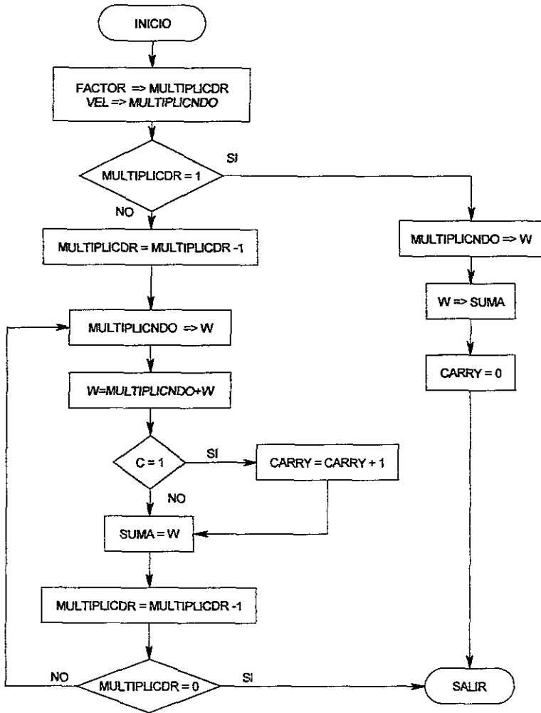
Figura 4.35. Diagrama de flujo de la subrutina de multiplicación.
