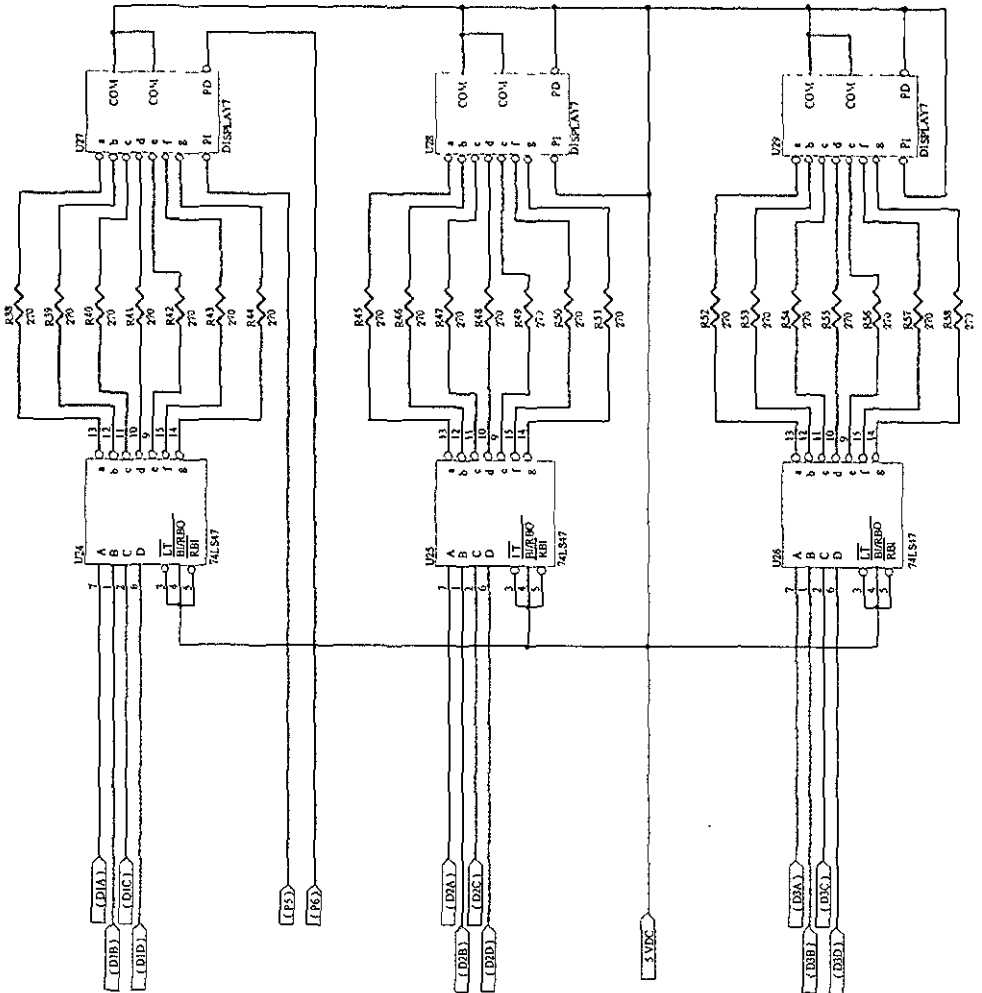
Figura 4.27. Diagrama eléctrico de la bomba de rodillos.
