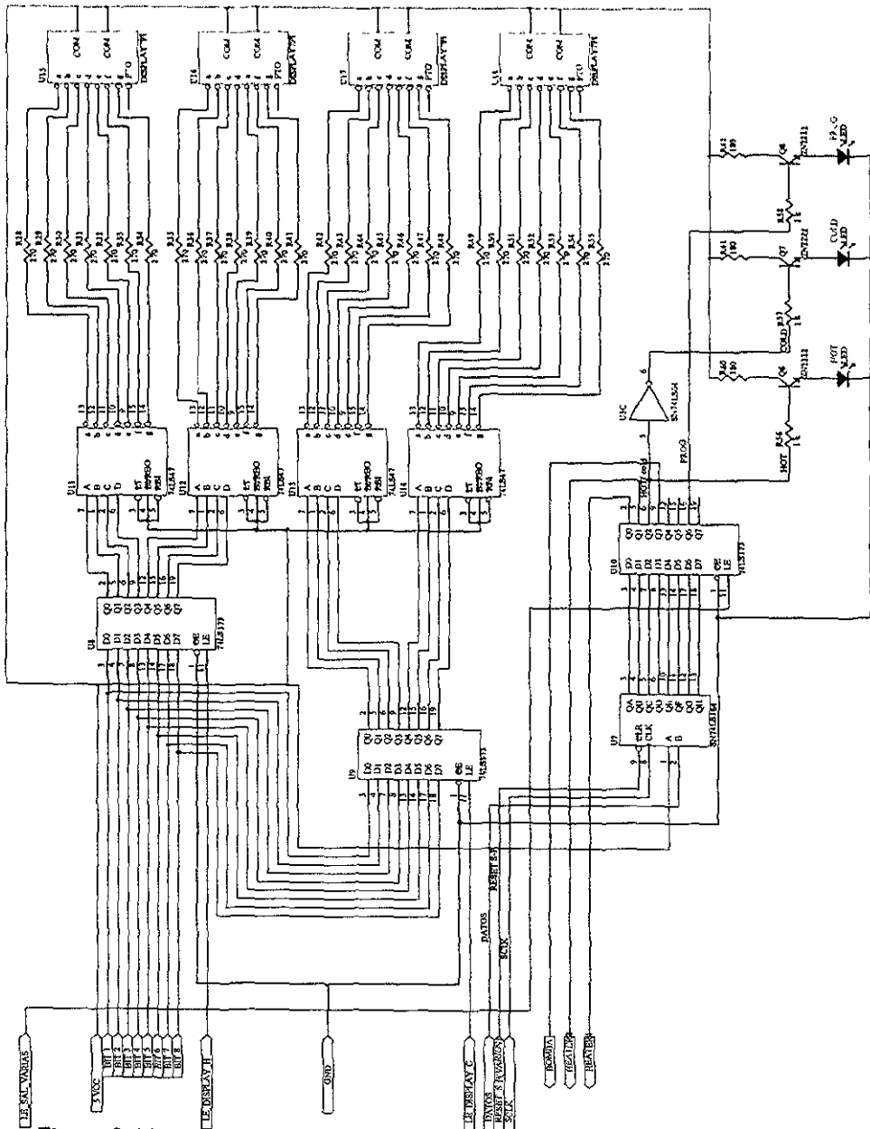
Figura 3.44. Diagrama eléctrico del intercambiador de temperatura. (Continúa).
