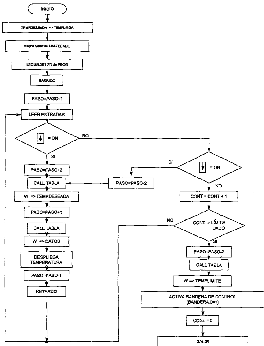
Figura 3.49. Diagrama de flujo de la subrutina de programación de la temperatura.
