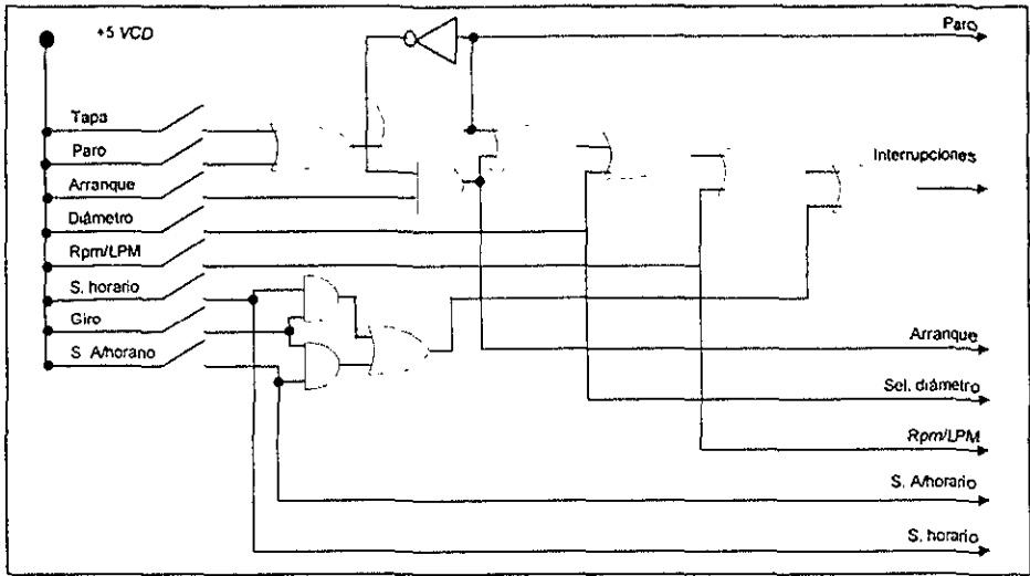
Figura 4.14. Circuito lógico para las entradas de control.
