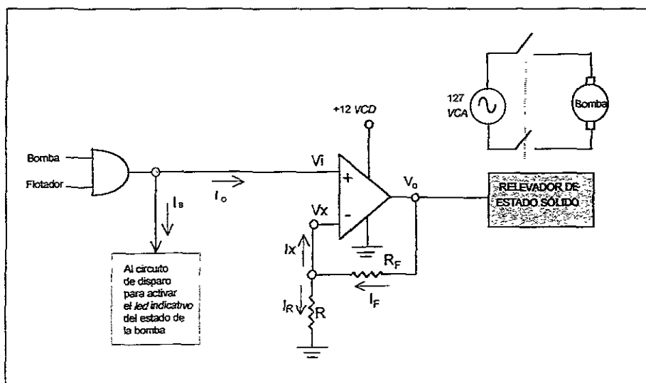
Figura 3.38. Circuito de control de activación de la bomba.
