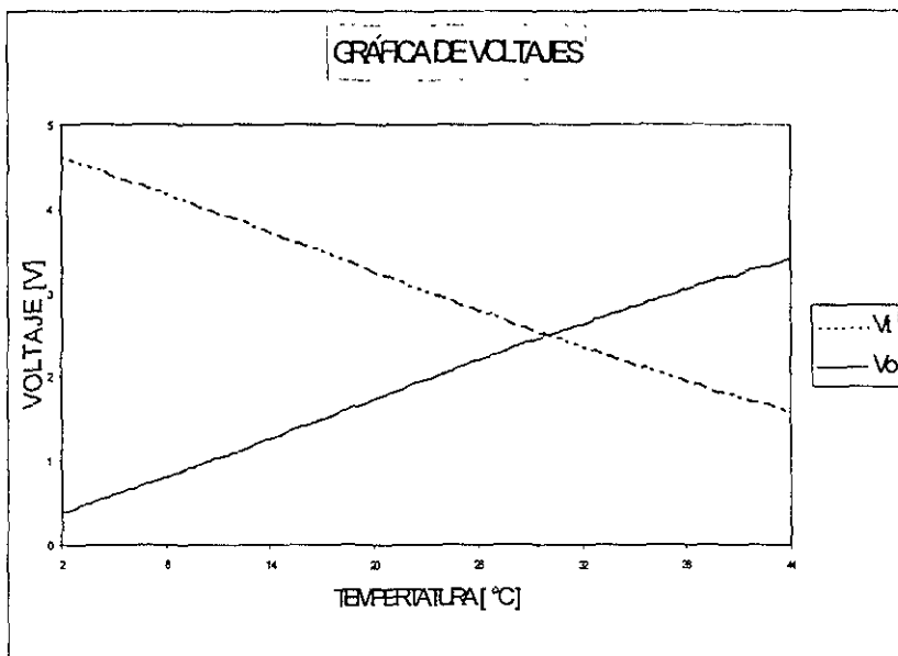
Figura 3.16. Gráfica comparativa de V_1 y V_0
