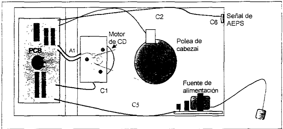
Figura 6.6. Vista inferior de la bomba de rodillos.
