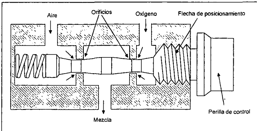
Figura 5.12. Módulo de proporción del mezclador de aire-oxígeno Sechrist.
