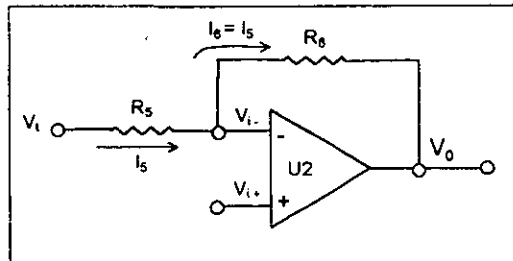
Figura 3.14. Circuito simplificado del voltaje de entrada a la terminal inversora del amplificador operacional U 2 .
