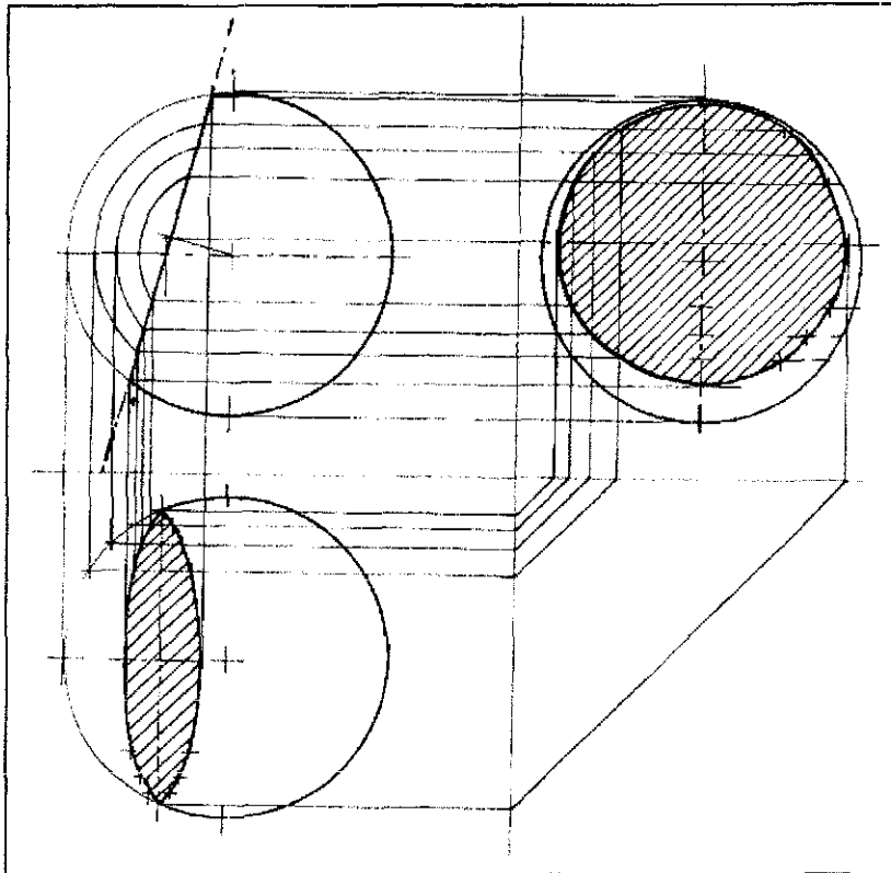
Sección de esfera con un plano perpendicular al P V e inclinado con respecto a los demás planos.
