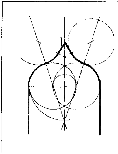
Arco conopial gótico o flamíngio
