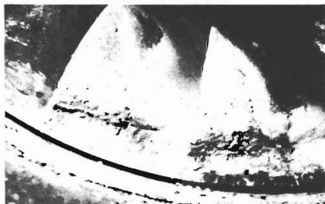
Figura 12.2. Desgaste por erosión producida por arena sobre los álaves de un rodete de bronce (Cortesía Allis Chalmers)
