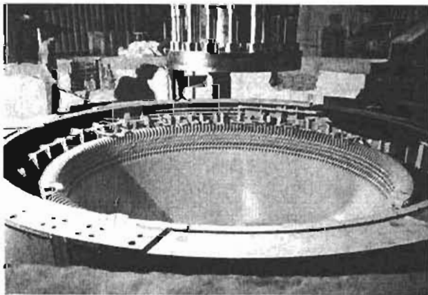
Estator
