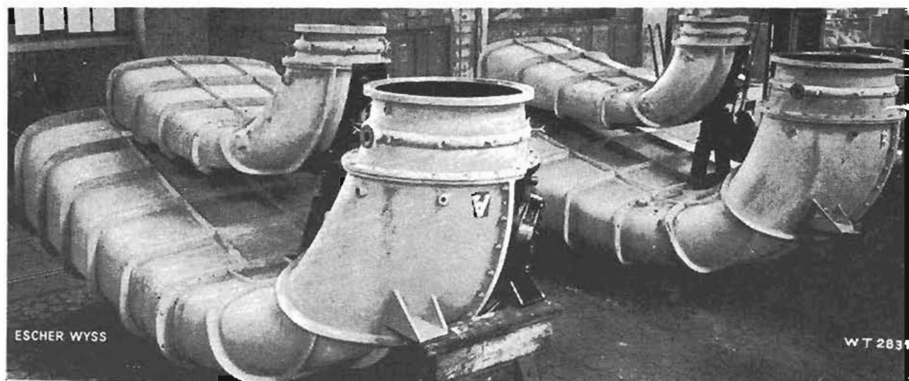
Figura 7.8. Tubos de desfogue para turbinas Kaplan (Cortesía Escher Wyss)
