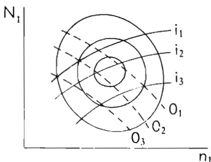
Figura 13.8. Curva característica de turbina Kaplan
