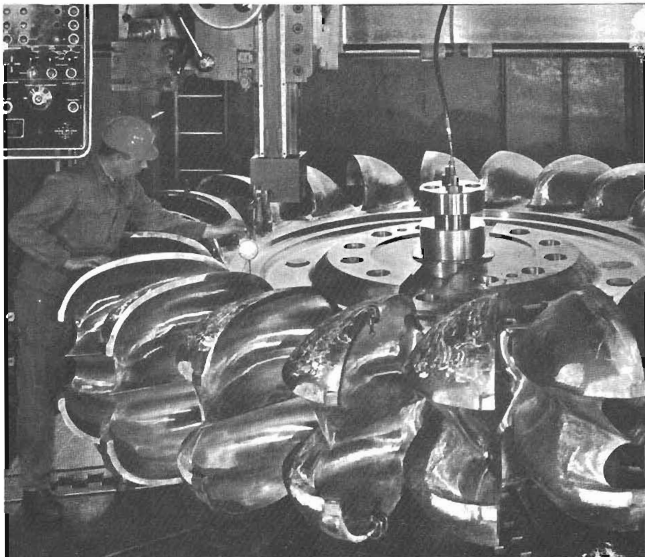
Figura 5.8. Moderna rueda Pelton en proceso de fabricación turbina de 6 chiftones para la planta de Castaic en Estados Unidos (Potencia 60.000 carga 321 m diámetro 3.75 m)
