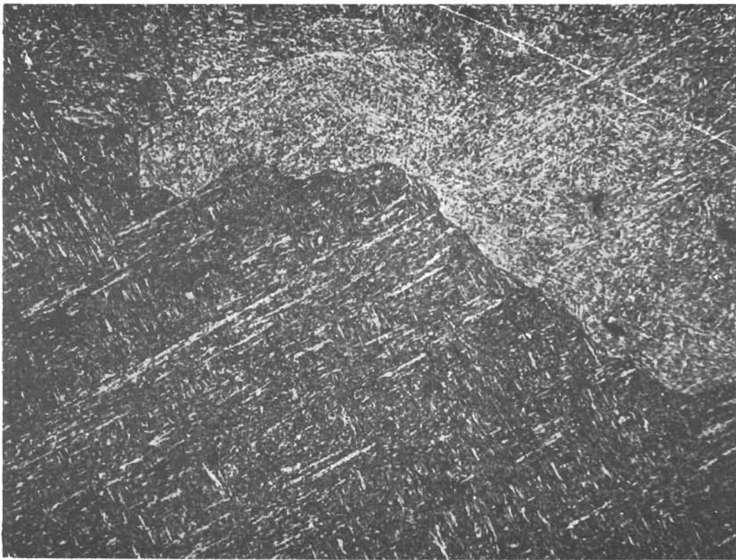
Figura 12.13. Microestructura (amplificación 100X) de un álabe de acero con 13% de cromo con buena resistencia a la cavitación. (Nótese la estructura martensítica y la distribución de los granos)
