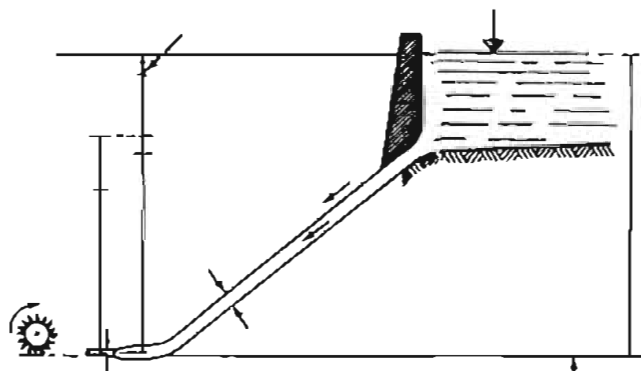
Figura 5.3. Esquema de flujo en las cangilonas
