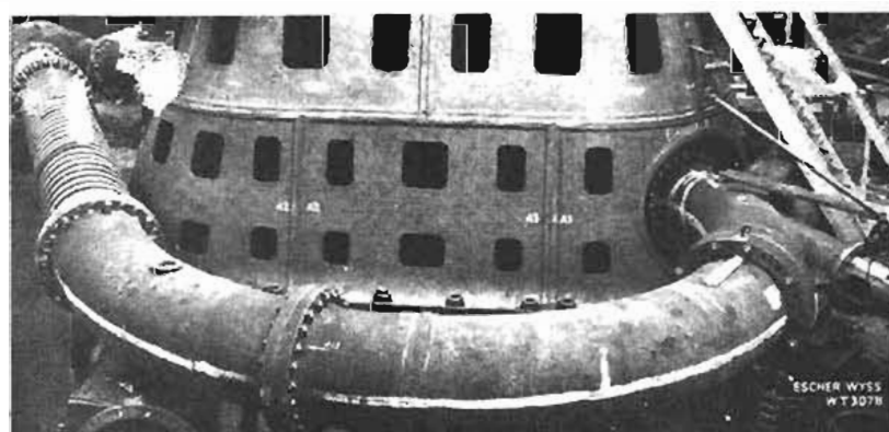
Figura 5.4. Muestra de dos de las agujas que controlan el flujo de las turbinas tipo Pelton de la planta de aberthasi (suiza).
