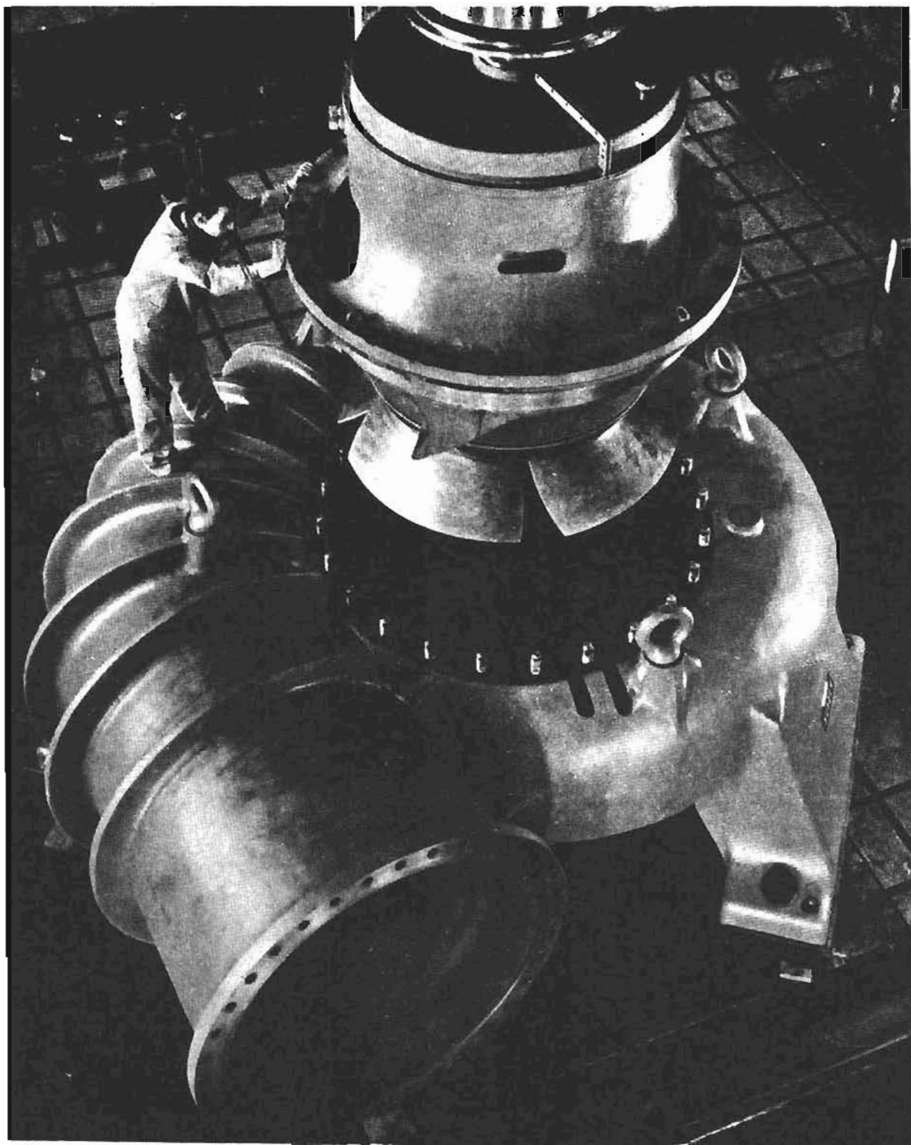
Figura 11.13. Tubo-Bomba semi-axial con paletas orientables para la central hidroeléctrica de acumulación por bombeo de Sesquile Colombia. Las potencias límites en servicio como bombas y como turbina son de 3855 CV y 4574 CV respectivamente a 450 r.p.m. Carga (32 a 39 m) Gasto 8000 y 12000 lts./seg. respectivamente (Cortesía Suizer)
