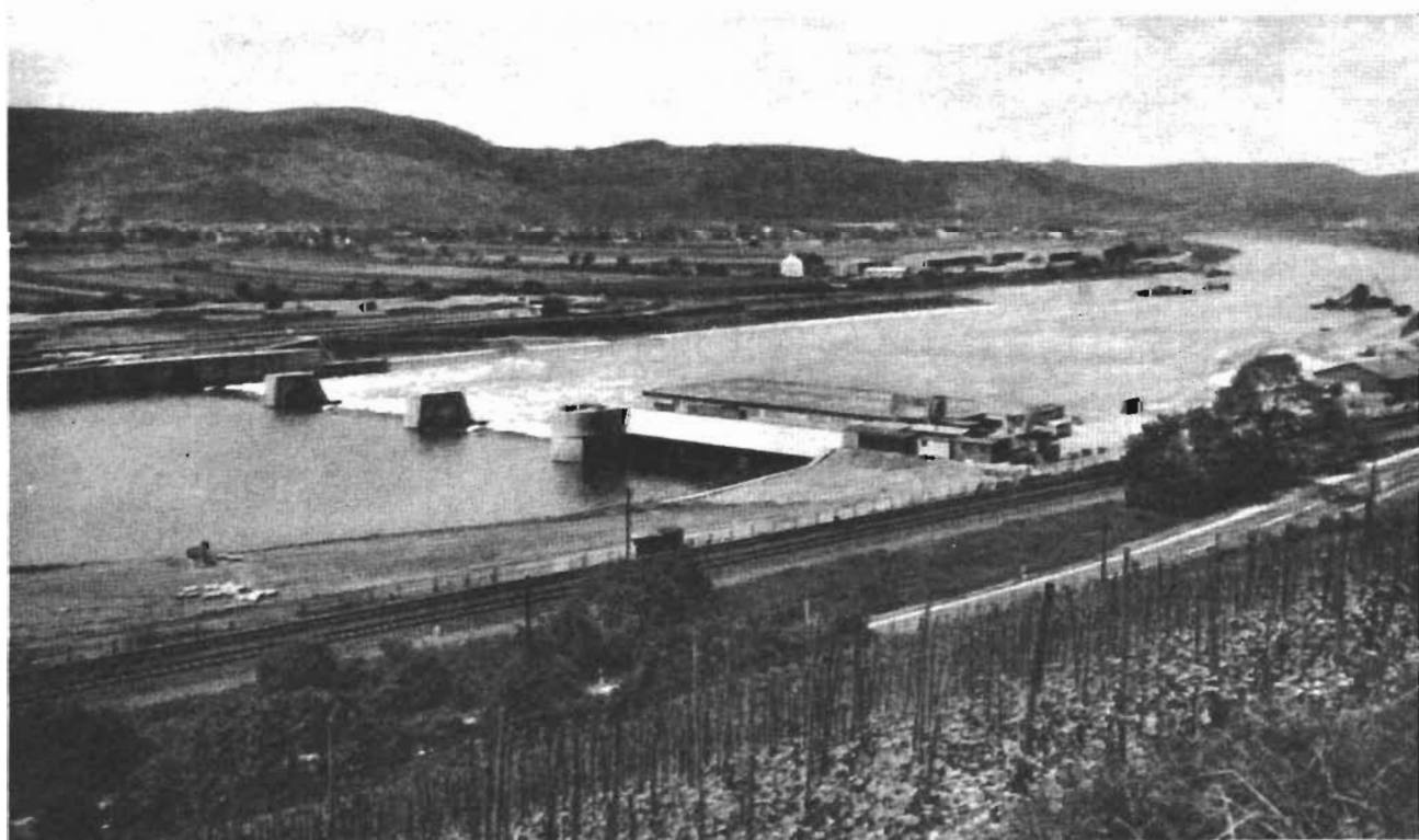
Figura 8.3. Planta hidroeléctrica de TRIER (Alemania) de baja carga con turbinas tubulares
