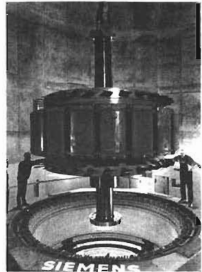
Rotor
