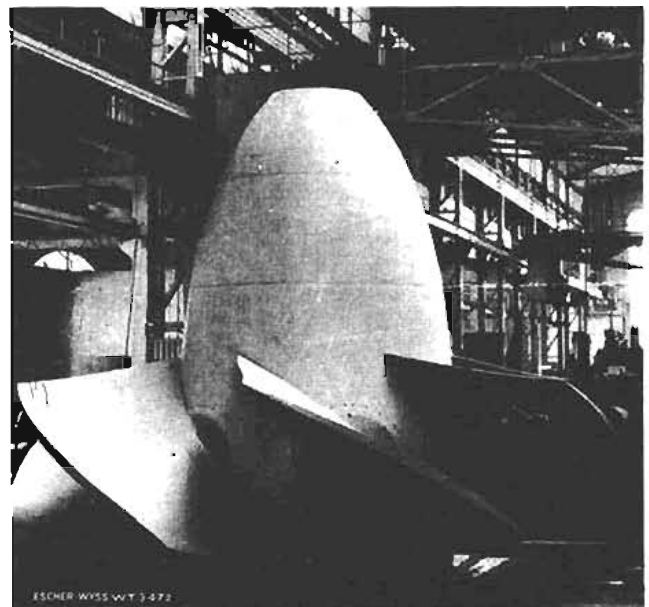
Figura 7.4. Una de las ruedas Kaplan, de unas 125 toneladas de peso, destinada a la central de Blondel del conjunto hidroeléctrico Bonzero-Mondragón. Foto tomada en talleres
