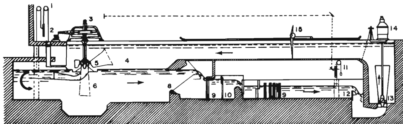
Figura 13.3. Diagrama de una instalación para pruebas de modelos Francis y Kaplan.
