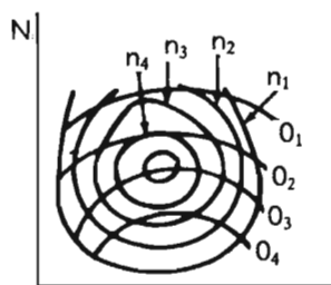
Figura 13.6. Curva velocidad-eficiencia.
