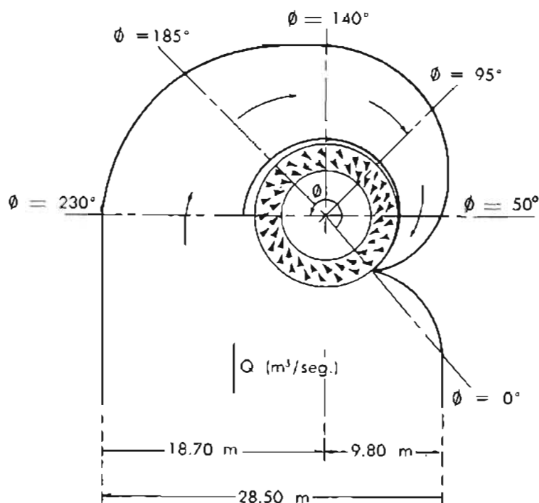
Figura 10.22. Espiral seccionada
