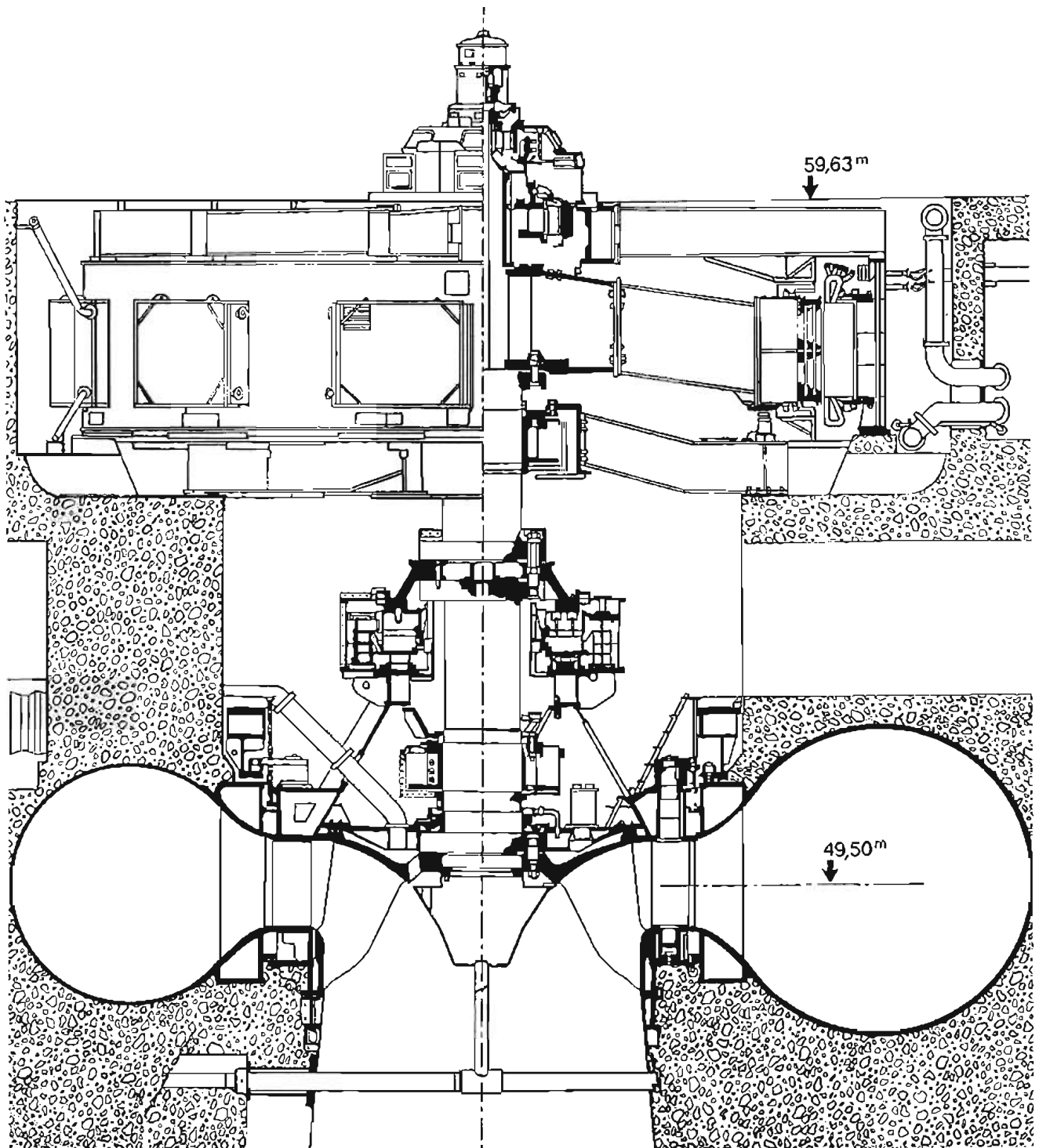
Figura 6.11. Corte seccional de las turbinas Francis de Infiernillo (México) (Cortesía NEVRPIC)
