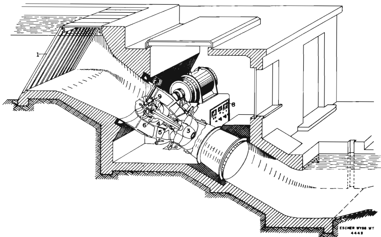
Figura 8.9. Diagrama de una turbina con transmisión cónica de engranes al generador.
