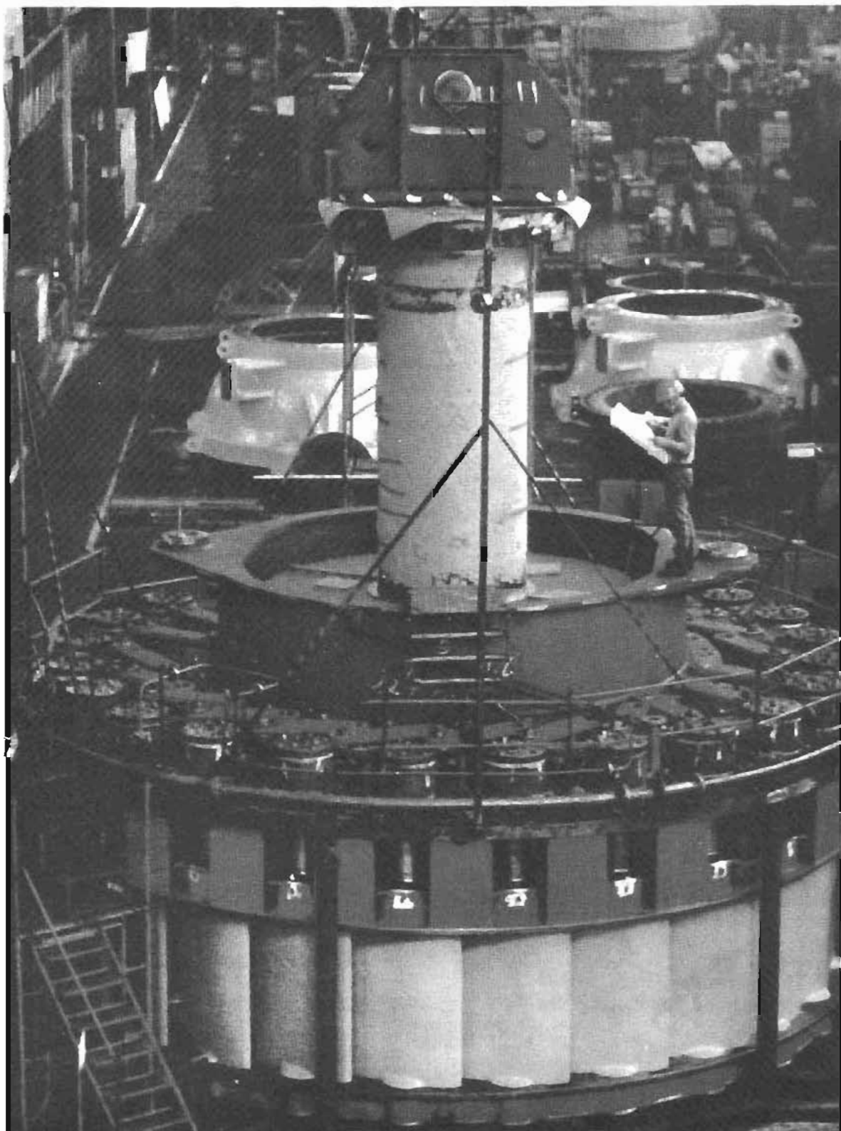
Figura 6.17. Rodete Francis para la planta hidroeléctrica de Guárico en Venezuela Potencia 270 mw Carga 139 m Velocidad 120 r.p.m.
