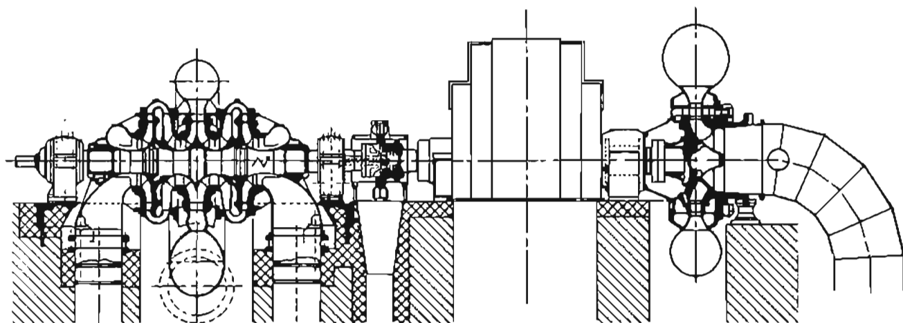
Figura 11.3. Arreglo horizontal de 3 máquinas (Planta Vianden Luxemburgo) Cortes(a), Escher Wyss.
