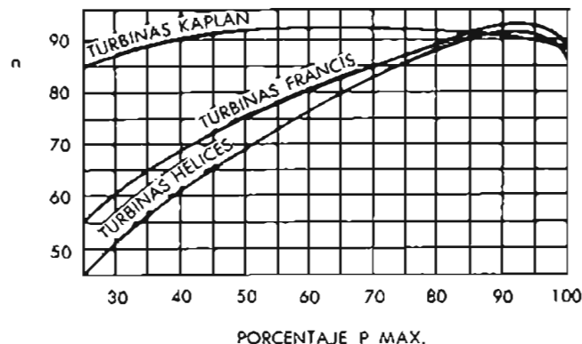
Figura 10.7. Curvas de eficiencia, según el porcentaje de P_{máx} de las turbinas.
