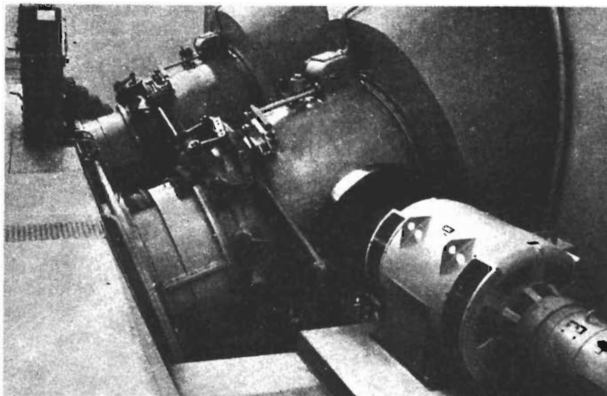
Figura 8.8. Planta típica con generador externo para la utilización económica de pequeños recursos hidroeléctricos Planta (Arlen Cotton Spinning Mill Riclasmgen/Radolfzell)
