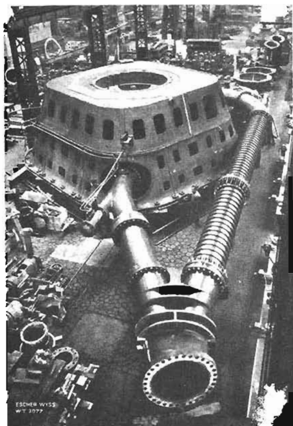
Figura 5.4. Muestra de dos de las agujas que controlan el flujo de las turbinas tipo Pelton de la planta de aberthasi (suiza).
