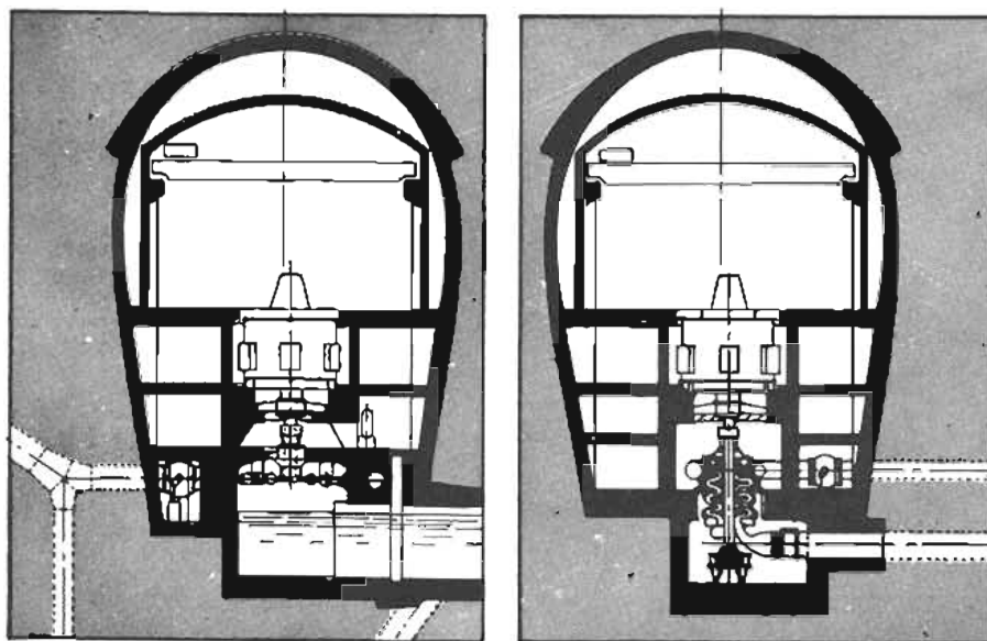
Figura 11.1. Planta con turbina y bomba separadas Turbina Pelton vertical H_{\text{máx}} = 1\,000\text{ m} P_{\text{máx}} = 150\text{ MW} n = 600\text{ r.p.m.} Bomba vertical de 4 pasos H_{\text{máx}} = 1\,015\text{ m} P_{\text{máx}} = 142.5\text{ MW} n = 600\text{ r.p.m.} (Cortesía, Escher Wyss)
