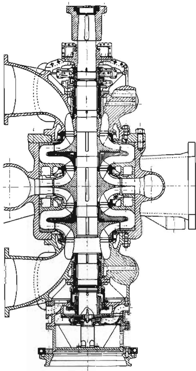
Figura 11.8. Arreglo de turbobomba reversible de 2 pasos de flujo, eje vertical
