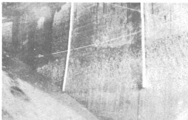
Figura 12.5. Otro ejemplo de un material clásicamente picoteada por el efecto de la cavitación. (Turbina Kaplan) (Cortesía Allis Chalmers)
