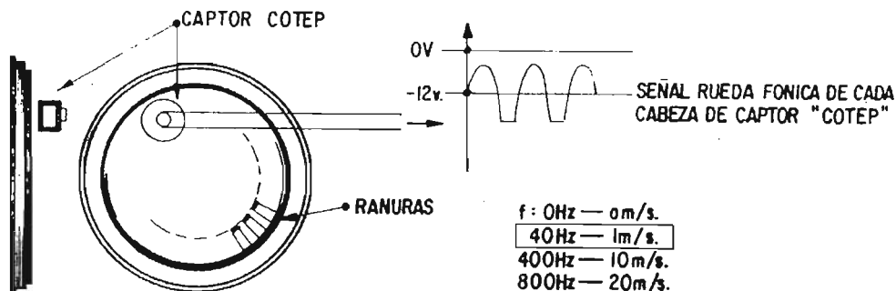
Figura IV-15 Rueda Fónica Y Captor COTEP
