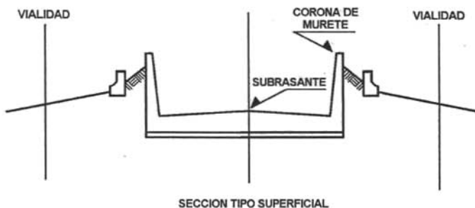
SECCION TIPO SUPERFICIAL
