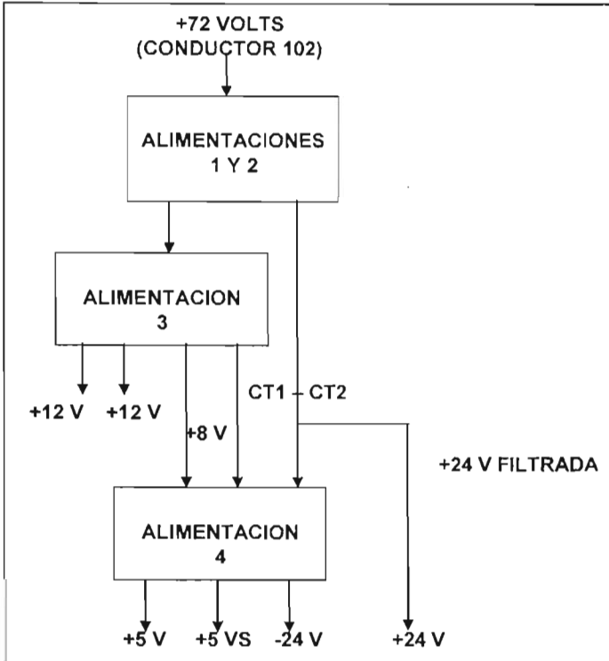
Figura IV-5 Alimentaciones 1, 2, 3 y 4 del block PA - CMC
