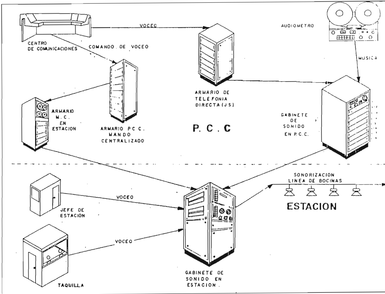
Figura IV-36 El Sistema De Sonorización
