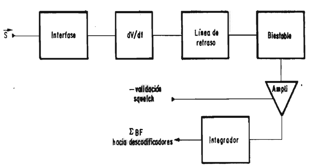
Figura IV-6 Principio Del Módulo Del Demodulador
