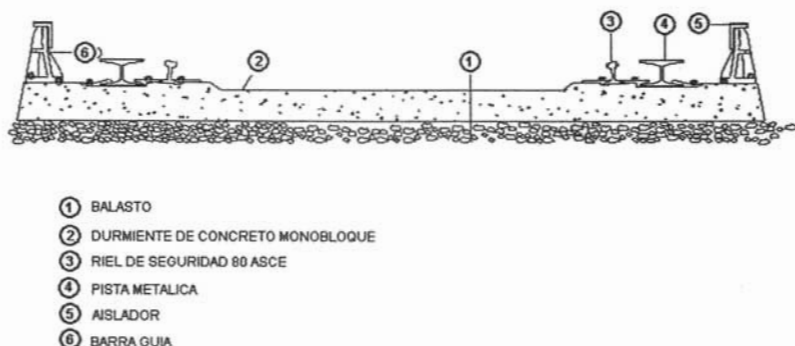
SISTEMA DE VIA SOBRE BALASTO CON DURMIENTES DE CONCRETO MONOBLOQUE
