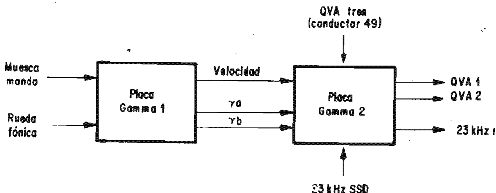
Figura IV-9 Principio De Los Módulos Gamma1 y Gamma 2
