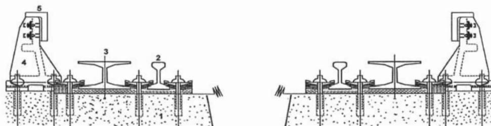
SISTEMA DE VIA SOBRE CONCRETO EN VIADUCTO
