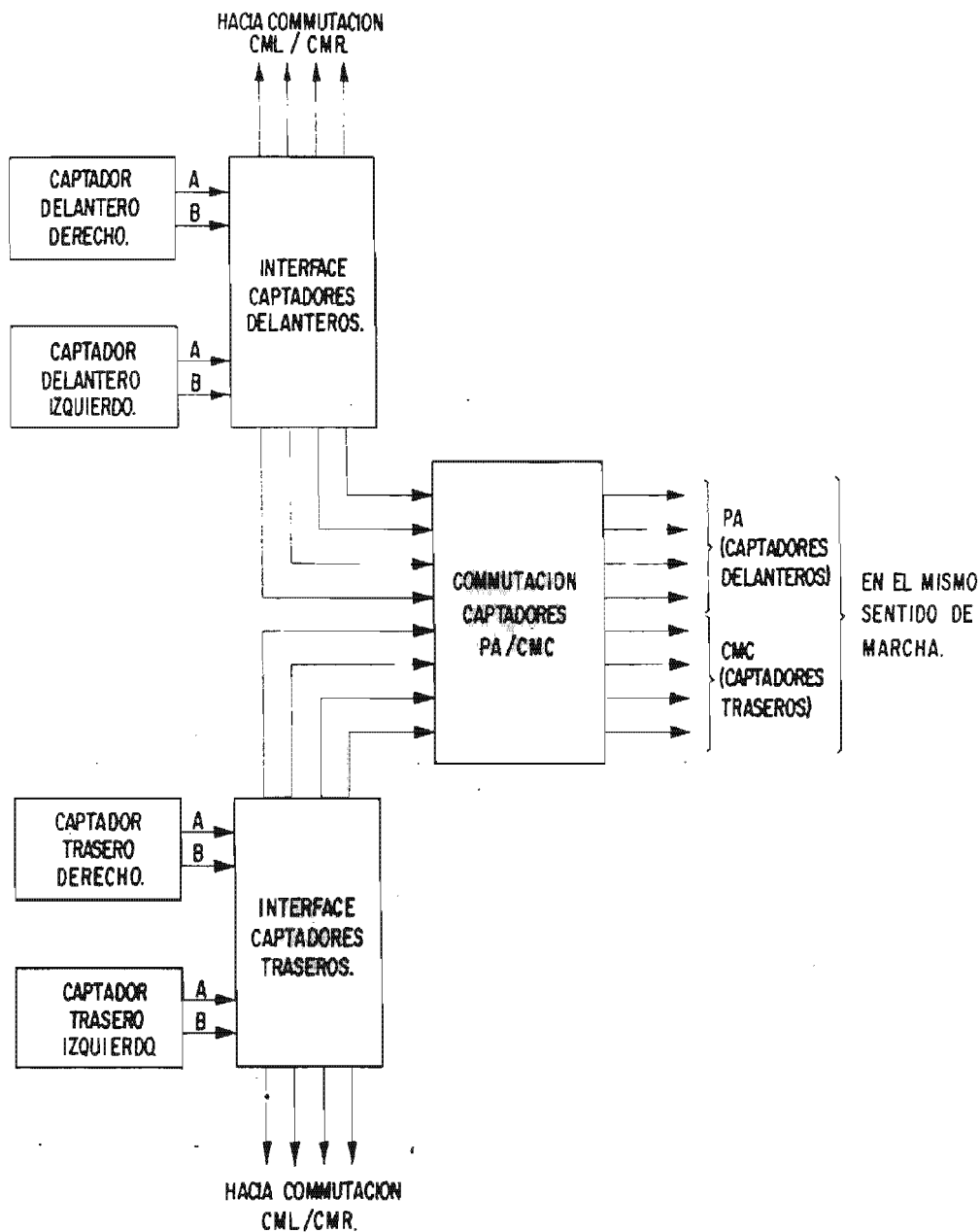
Figura IV-13 Principio De La Conmutación De Los Captore
