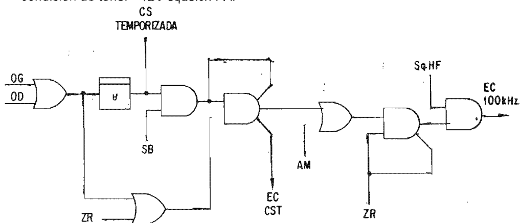
Figura IV-10 Diagrama Del Módulo Energía Cable
