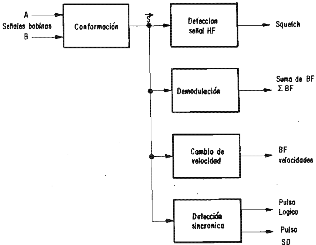
Figura IV-11 Módulo De Captación PA – CMC
