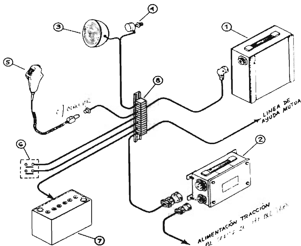
Figura IV-34 Sinóptico De Trenes
