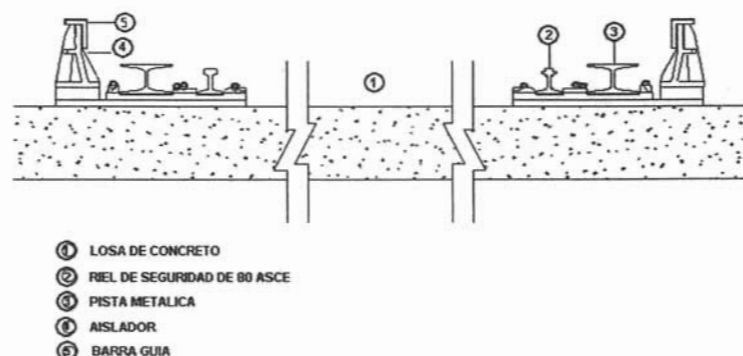
SISTEMA DE VIA SOBRE LOSA DE CONCRETO
