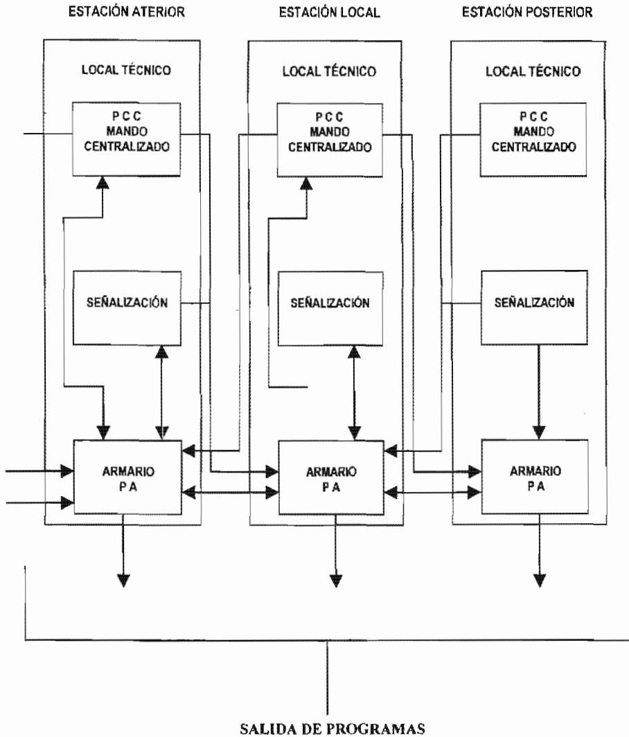
INTERCONEXIONES DE LOS ARMARIOS DE PA ENTRE SI Y CON OTROS EQUIPOS
