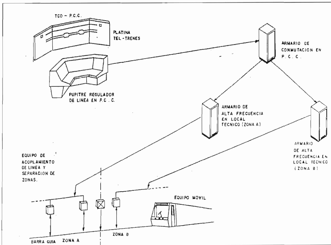
Figura IV-33 Telefonía De Trenes
