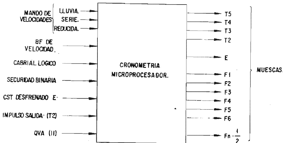
Figura IV-12 Módulo De La Cronometría
