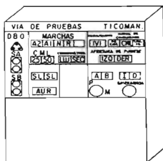
ARMARIO VIA DE PRUEBAS.
