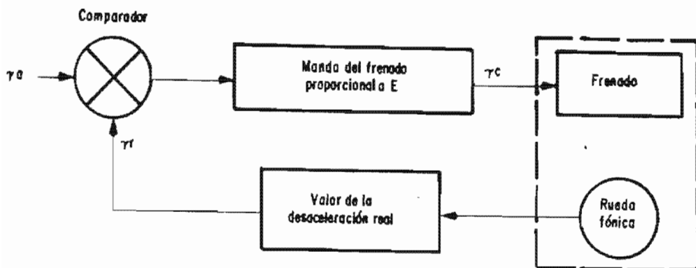
Figura IV-8 Principio Del Módulo Gamma1
