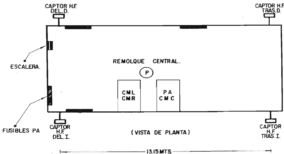
Figura IV-16 Disposición De Los Bloques y Captores del P. A. Embarcado
