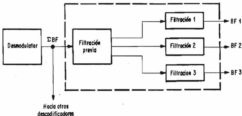
Figura IV-7 Principio Del Módulo Decodificador
