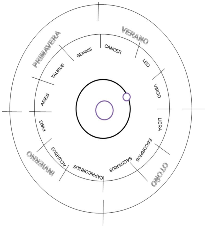
Figura 2. El zodiaco.
