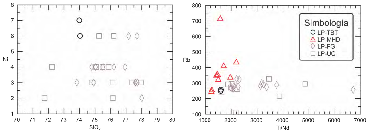
Figura 20. Diagramas binarios de elementos traza, normalizados en base anhidra y en ppm, SiO 2 en wt%. La simbología corresponde a la Figura 2. Nomenclatura: LREE (Light Rare Earth Elements), HREE (Heavy Rare Earth Elements), HFSE (High Field Strength Elements), LILE (Large Ion Lithophile Elements).
