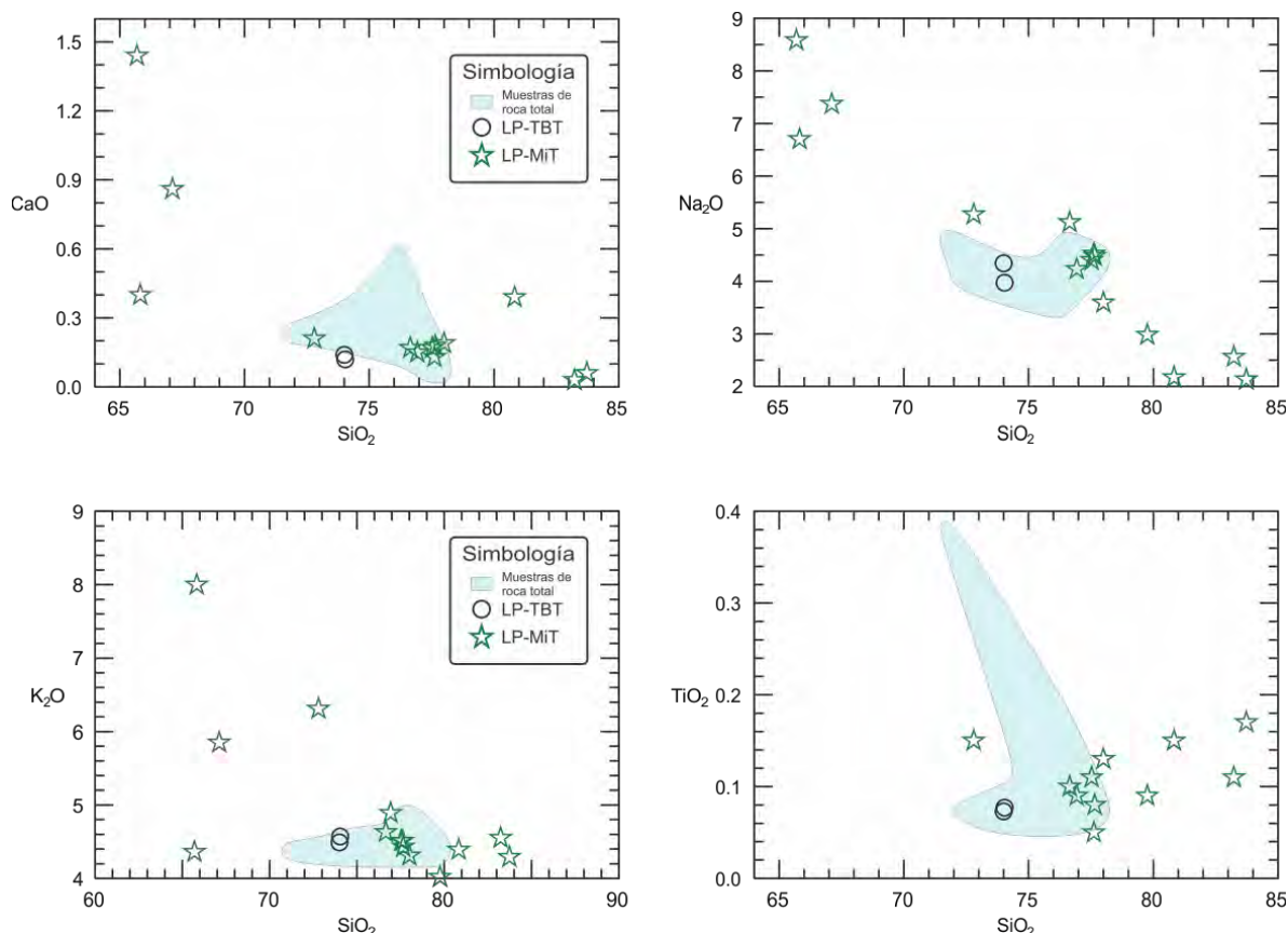
Figura 19. Diagramas binarios de elementos mayores normalizados a base anhidra de las muestras estudiadas. Claves de la simbología el área de color azul corresponde a las muestras de roca total de La Primavera publicadas por Cruz-Lara (2015), Gómez-Álvarez (2015) y Mahood (1981). LP-TBT) Pómez Toba Tala. LP-MiT) Inclusiones de Vidrio.
