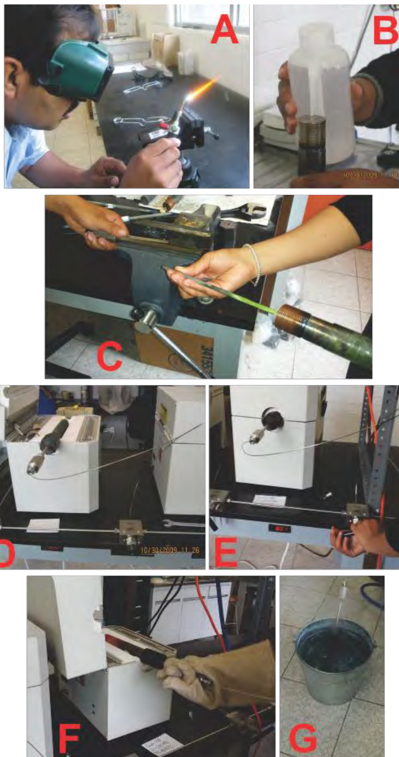
Figura 14. Fotografías de los pasos para realizar un experimento. A) Soldar la cápsula una vez llena con los reactivos y agua. B) Colocar la cápsula en el tubo de presión y llenar con agua. C) Colocar el tubo de Níquel para la línea de presión. D) Situar la línea de presión en el horno. E) Establecer la presión y temperatura a la cual se correrá el experimento. F) Terminado el tiempo del experimento desconectar la línea de presión y retirar el horno. G) enfriamiento súbito para preservar las condiciones del experimento.
