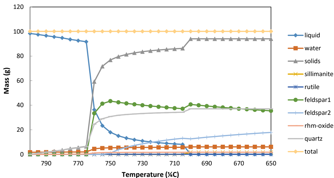
Figura.23. Gráfica de la secuencia isobárica con la composición de TTiM-07 (tabla 2) a una presión de 150 MPa, con un \Delta T=10 de 800 a 650 °C. generada a partir de la herramienta Rhyolite-MELTS.
