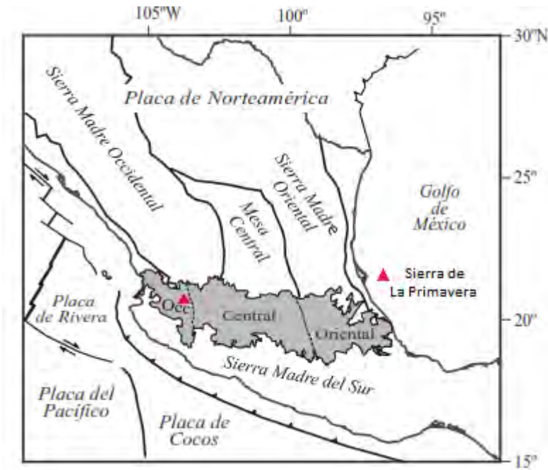
Figura 2. Ubicación de la Faja Volcánica Transmexicana (en gris), de las principales provincias geológicas de México y de las placas tectónicas actuales. También se muestra la ubicación de los tres sectores de la FVTM, la ubicación de la Sierra de La Primavera (Tomado/Modificado Gómez-Tuena et al., 2005).
