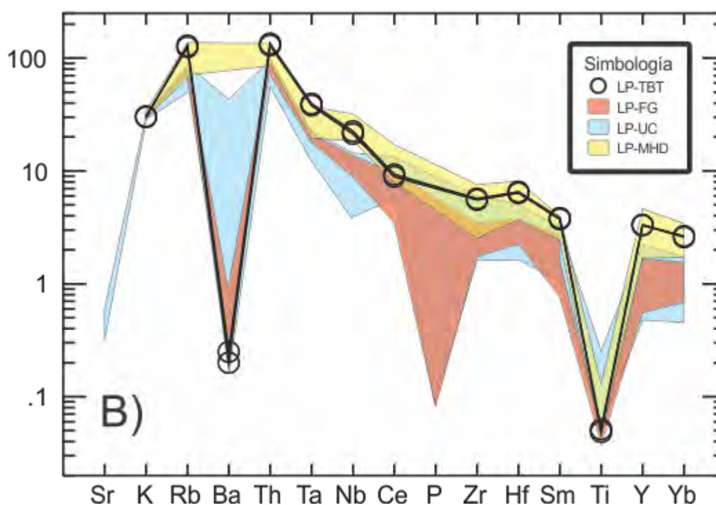
Figura 21. Diagramas spider A) distribución de elementos normalizados respecto a la condrita (Sun & McDonough, 1989). B) distribución de elementos normalizados respecto al MORB (Pearce, 1983). Simbología. LP-TBT) muestras de pómez de la Toba Tala. LP-FG) muestras de roca total de los domos Collí y El Tajo publicadas por Gómez-Álvarez (2015). LP-UC) muestras de roca total del domo San Miguel publicadas por Cruz-Lara (2015). LP-MHD) muestras de roca total de la caldera de La Primavera publicados por Mahood (1981).
