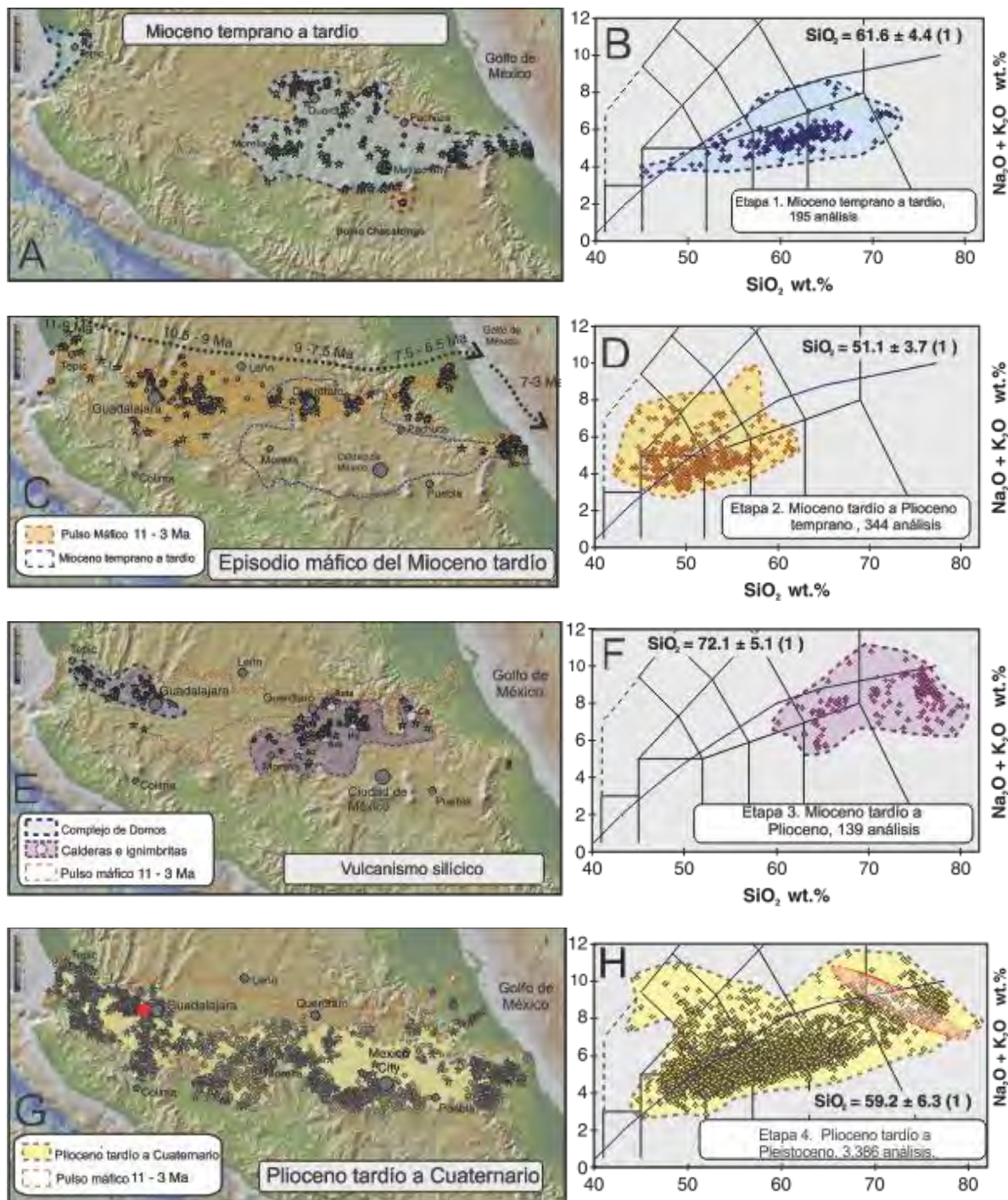
Figura 3. Distribución del vulcanismo en cada etapa y diagrama TAS asociado. A) Primera etapa del Mioceno temprano al tardío. B) Los magmas de la primera etapa corresponden a la serie sub-alcalina desde basalto a riolita. C) Distribución espacial del pulso mafico (área naranja) al oeste de la primera etapa. D) Clasificación de las rocas de la segunda etapa. E) Distribución del vulcanismo silícico (calderas e ignimbritas). F) La mayoría de las muestras de la tercera etapa se clasifican como riolita. G) Distribución espacial de la cuarta etapa, se observa una mayor distribución con respecto a las demás etapas de la FVTM, la caldera de La Primavera se representa por el círculo rojo. H) Las muestras de la cuarta etapa muestran una mayor variación en la composición de los magmas de la FVTM, el área de color rojo representa la clasificación de las MI y muestras de roca total de La Primavera. (Tomado/Modificado de Ferrari et al, 2011)
