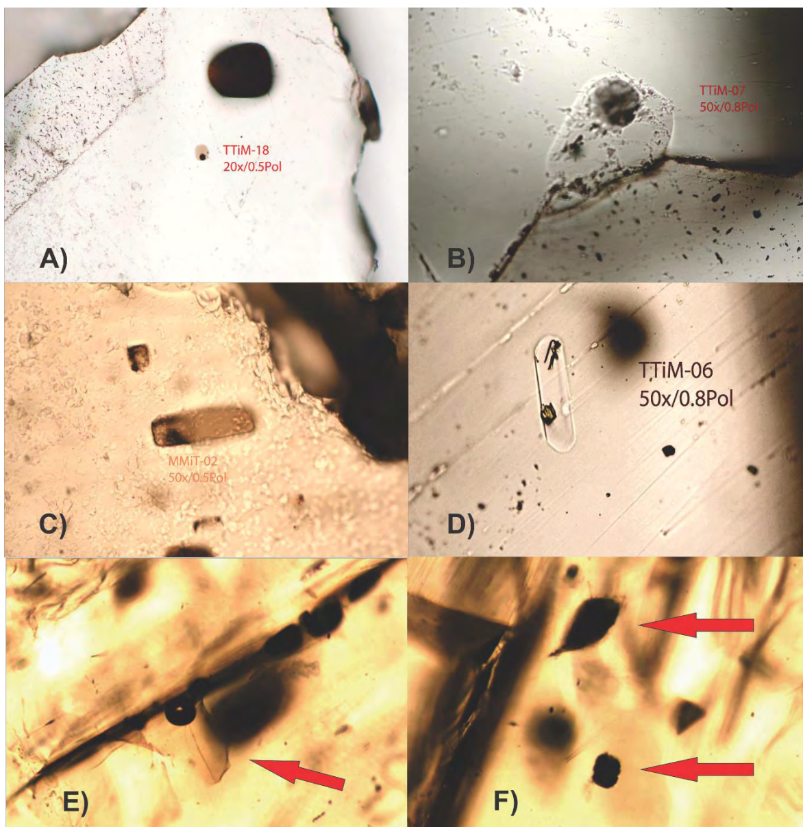
Figura 22. Fotomicrografías de las MI analizadas en el presente trabajo (A, B, C y D) y ejemplos de MI con procesos post-cristalización (PEC), las cuales no fueron analizadas en el presente trabajo (E, F). A) Aspecto de las MI en relación al tamaño del cristal que las contiene B) MI del grupo 2 totalmente expuesta con la burbuja de CO 2 reventada. C) MI del grupo 1, éste grupo se caracteriza por las tonalidades marrones de las MI. D) MI del grupo 1 con posibles cristales hijos, éstos son de tonalidades verdes. E) MI afectada por PEC, en donde la morfología de la MI se ve afectada por la fractura del cristal host. F) MI desvitrificadas
