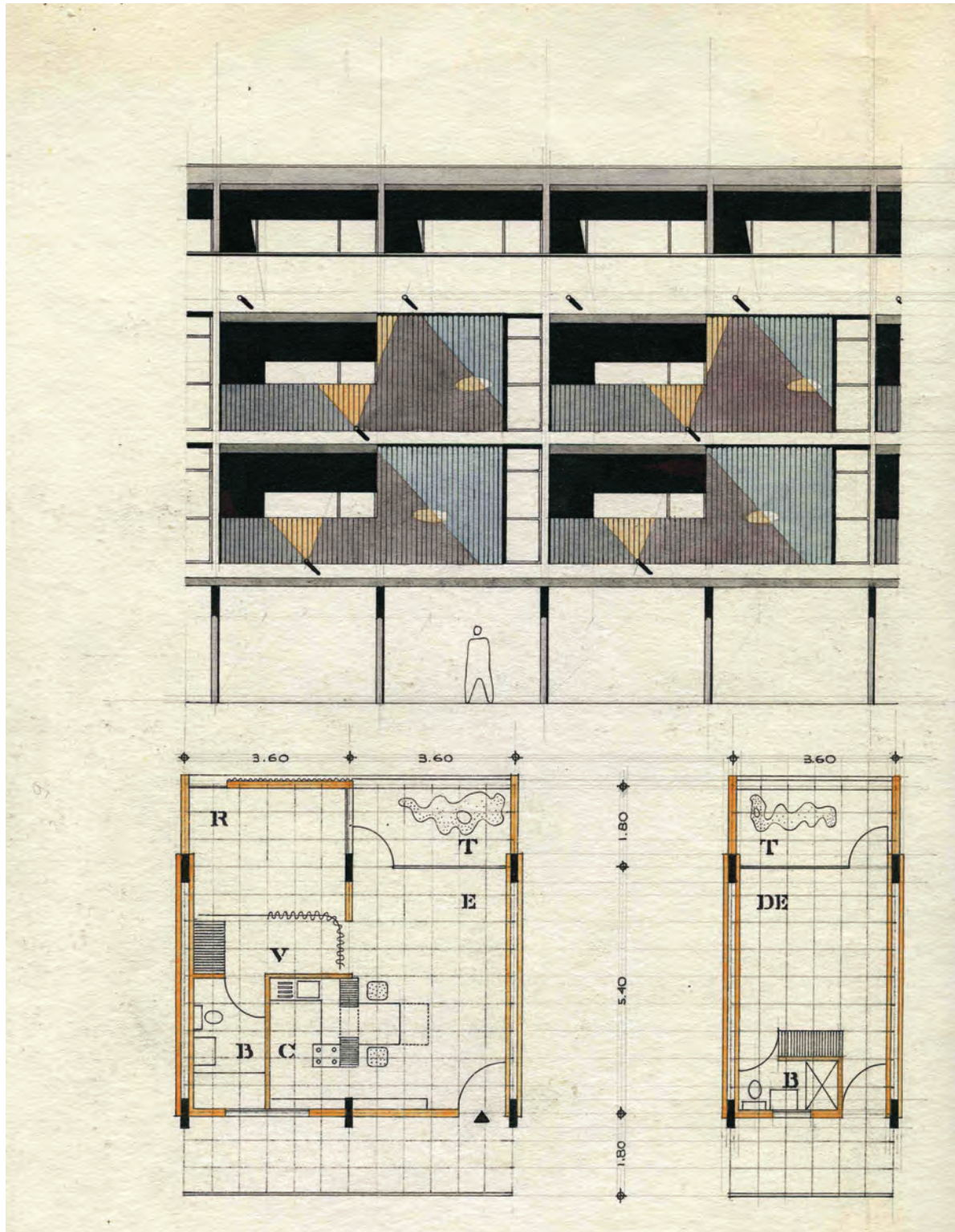
Multifamiliar, aproximaciones. Sección de fachada; planta depto. A y B con módulos. AAM
