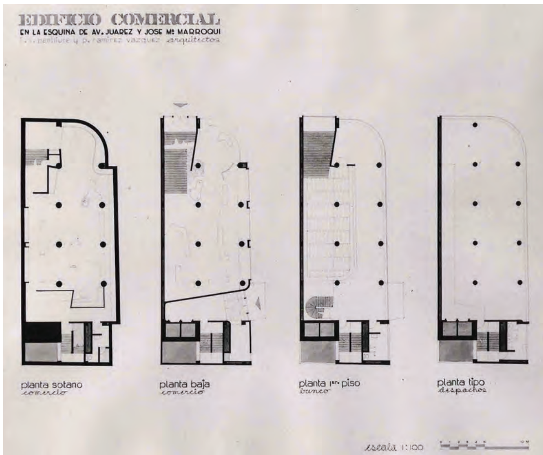
Edificio comercial. Plantas arquitectónicas. FMB
