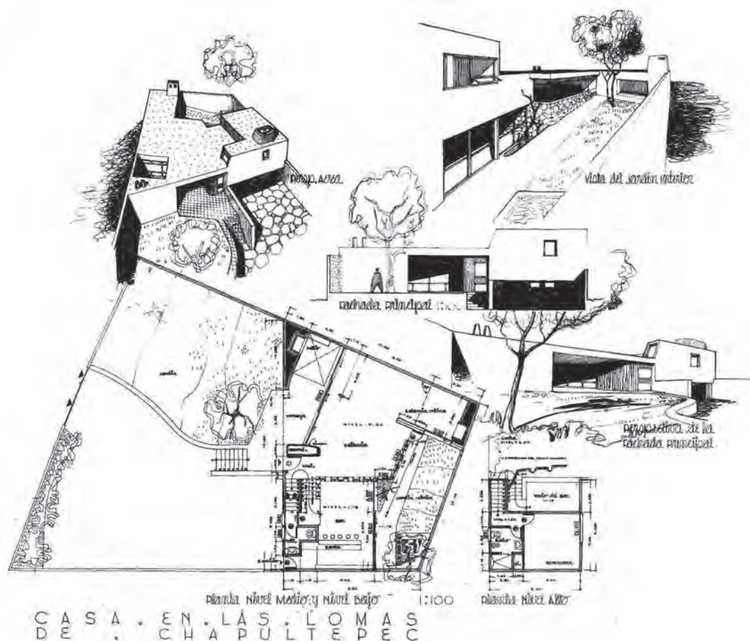
Casa en las Lomas, lámina. Plantas, fachada y perspectivas A-PRV
