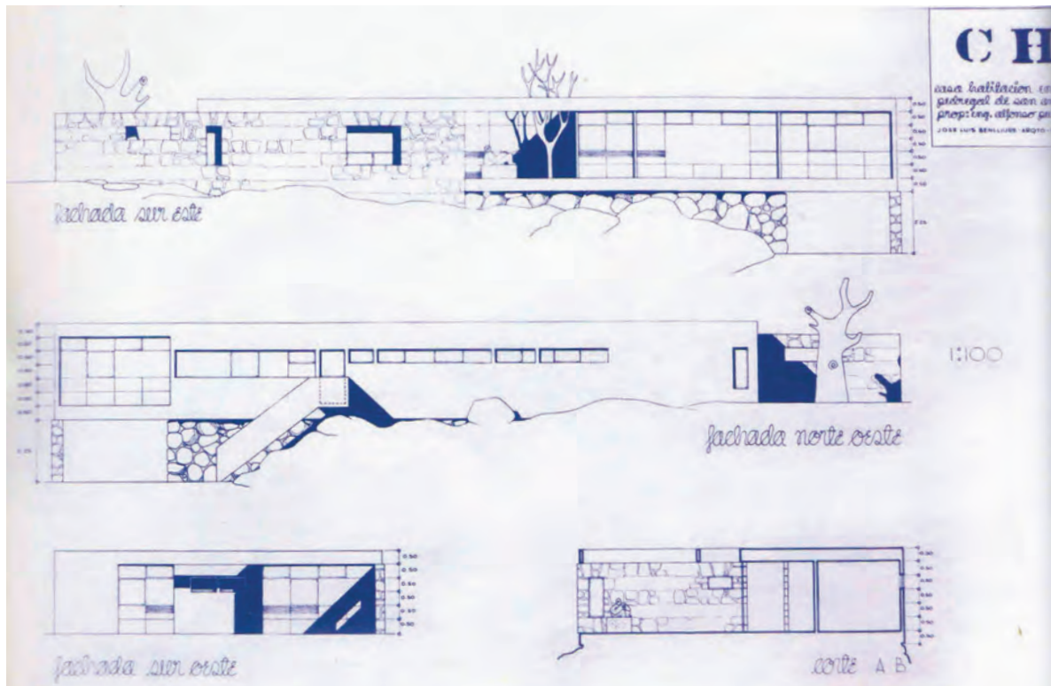
Casa Pulido. Fachadas y sección. ABB (publicado por RLR)
