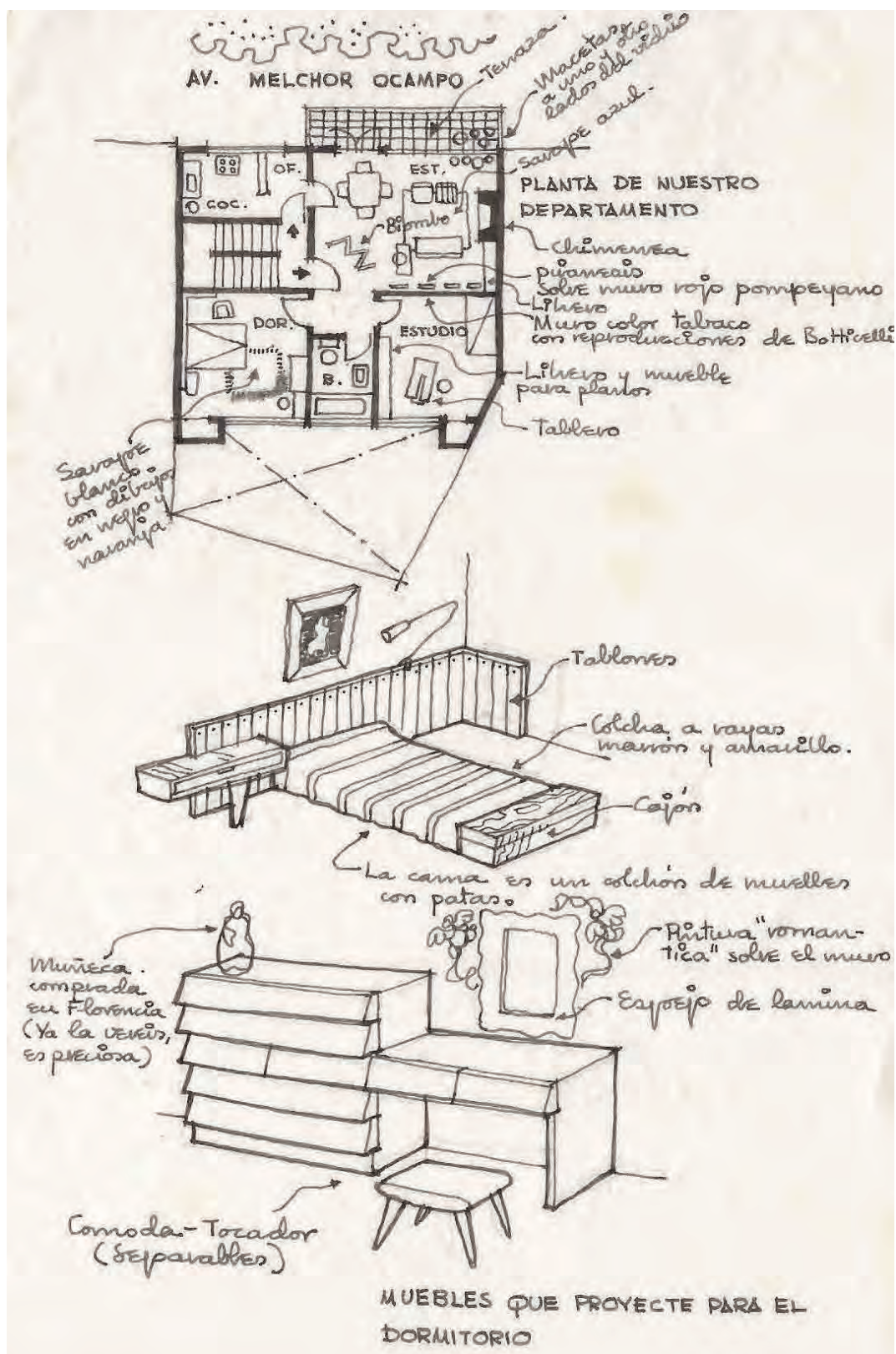
Diseño interior del departamento en Melchor Ocampo, aproximaciones. Planta y mobiliario. FMB (correspondencia).
