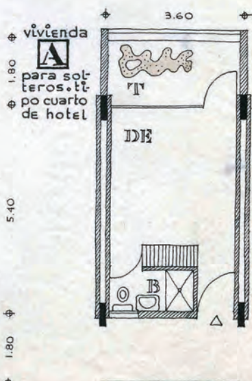
Multifamiliar, aproximaciones. Sección de fachada; planta depto. A y B . AAM
