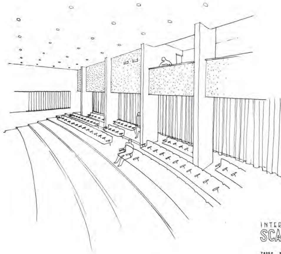
SCACZMPV, lámina 10 (detalle) y lámina 17. Fachada este y perspectiva interior del auditorio. A-PRV
