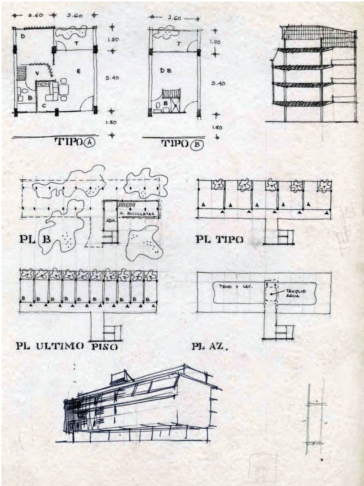
Multifamiliar, aproximaciones. Planta depts. A y B; planta baja, tipo, último piso y azotea; sección transversal; perspectiva. AAM
