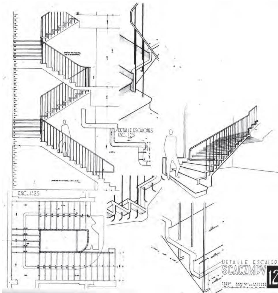
SCACZMPV, láminas 11 y 12. Secciones transversales y detalle de la escalera principal. A-PRV
