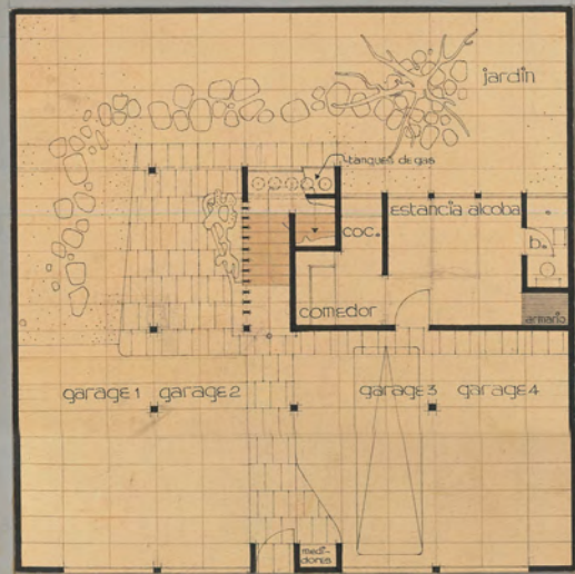
planta baja
