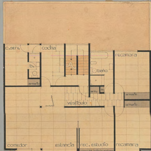
planta tipo
