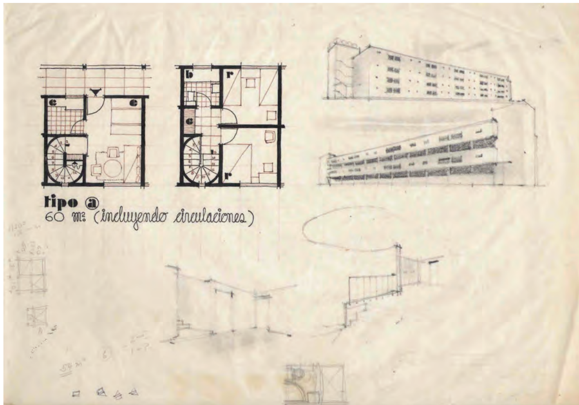
Multifamiliar, aproximaciones. Planta depto. A; perspectivas exteriores (fachadas) e interiores (depto. A); esquemas. FMB
