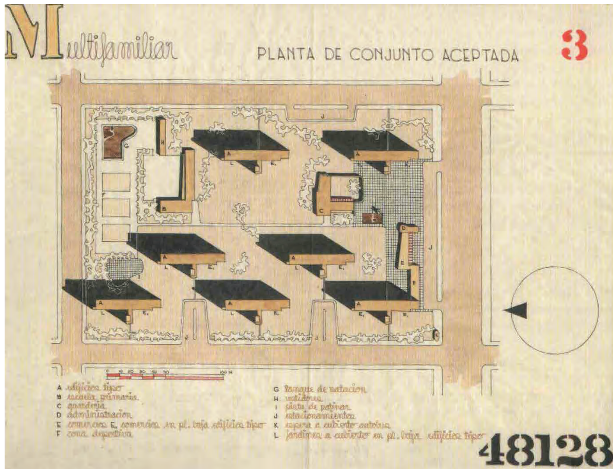
Multifamiliar, concurso entregado, lámina 3. Planta de conjunto aceptada. ABB (publicado por RLR)
